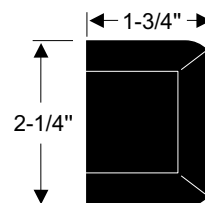
END CAP
